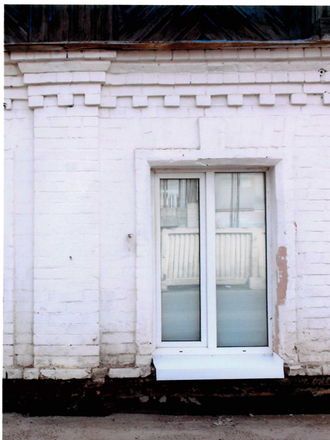
Видовая точка № 6. Окно 1-го этажа главного фасада. Элементы декора (профильный пояс с сухариками, обрамления окон с замковым камнем, пилястра).
